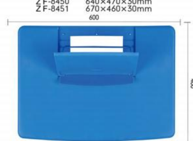
Z F-8196 600×400×18mm
