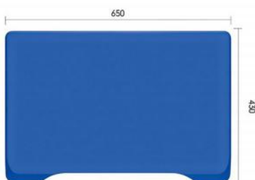
Z F-8317 650×430×30mm Z F-8447 600×400×30mm Z F-8448 660×450×30mm
